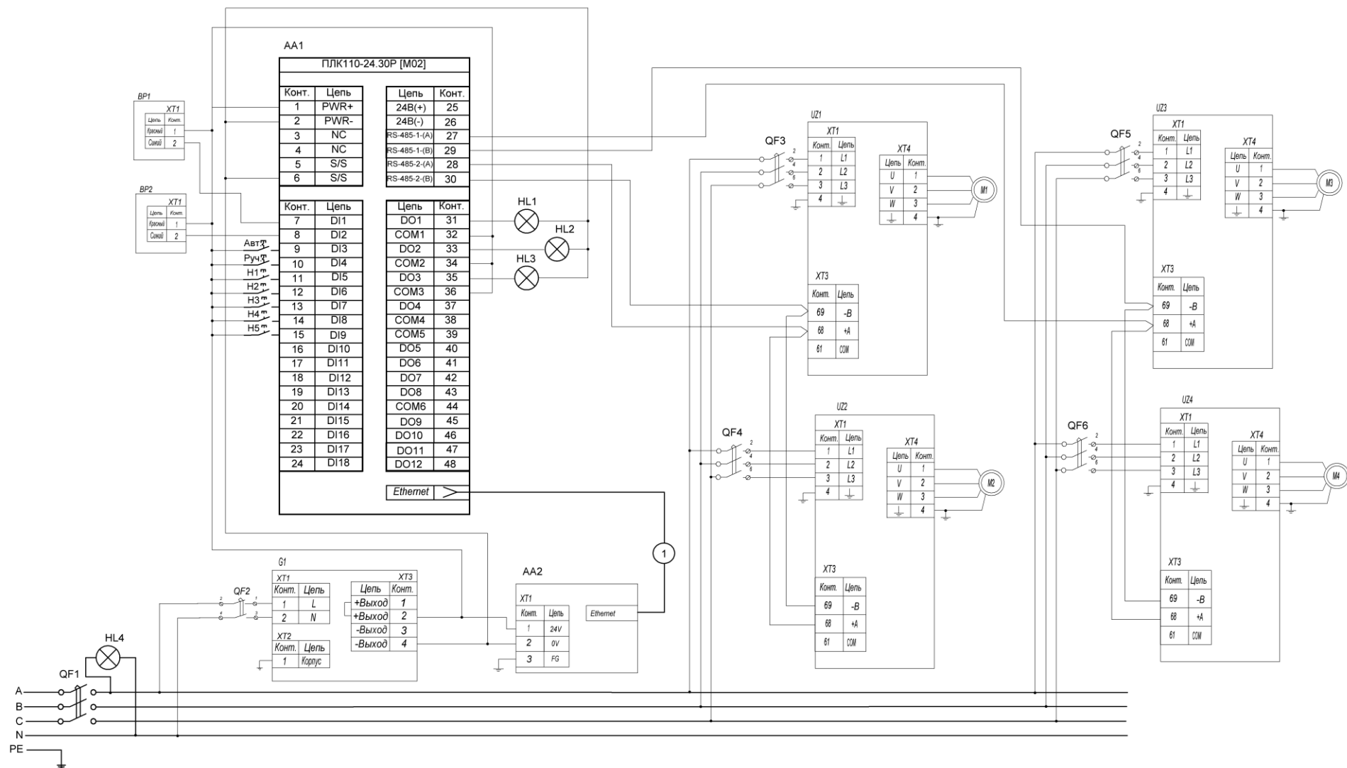
Рисунок 4.5 – Электрическая схема подключения
