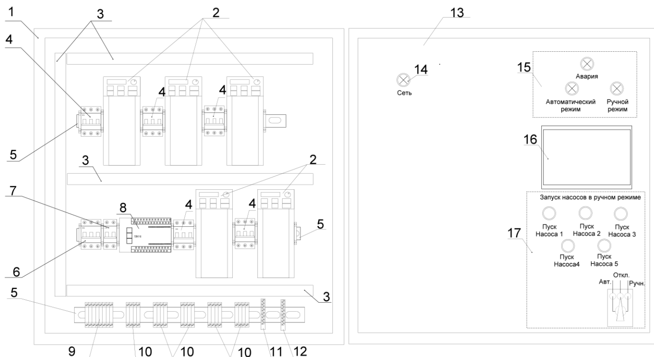
Рисунок 4.1 – Шкаф управления станцией пожаротушения *:
