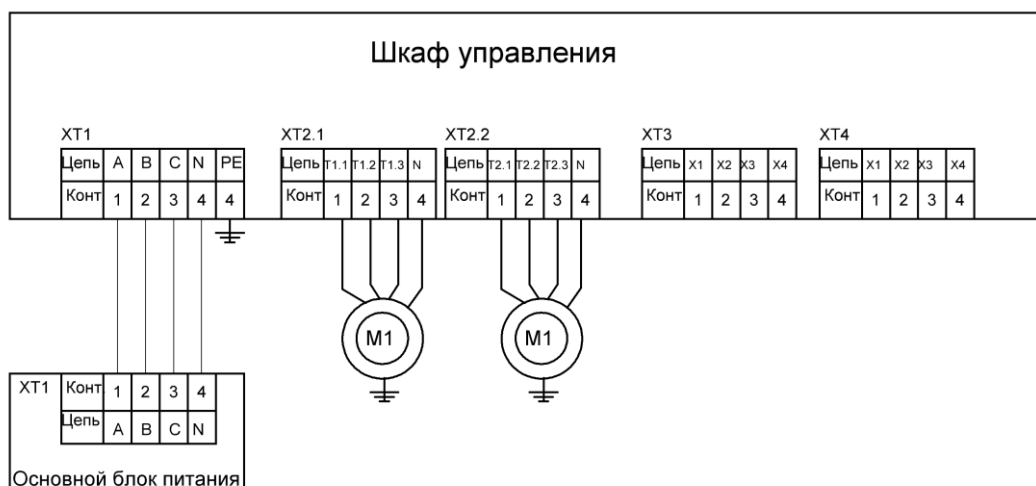
Рисунок 4.2 – Принципиальная схема внешних электрических подключений шкафа управления*: XT1 – клемма подключения внешнего питания шкафа (фазы А,В,С,нейтраль N, клемма заземления PE); XT2.1, XT2.2 – клеммы подключения двигателей управления; XT3,XT4 – клеммы подключения к устройствам управления (состав клемм зависит от выбранного устройства).
