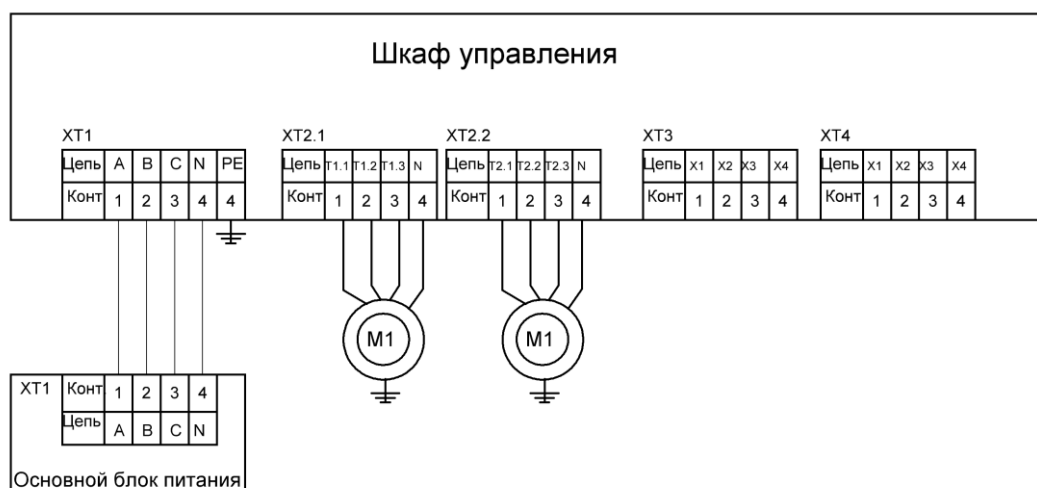
Рисунок 4.2 – Принципиальная схема внешних электрических подключений шкафа управления*: XT1 – клемма подключения внешнего питания шкафа (фазы A,B,C,нейтраль N, клемма заземления PE); XT2.1, XT2.2 – клеммы подключения двигателей управления; XT3,XT4 – клеммы подключения к устройствам управления (состав клемм зависит от выбранного устройства).
