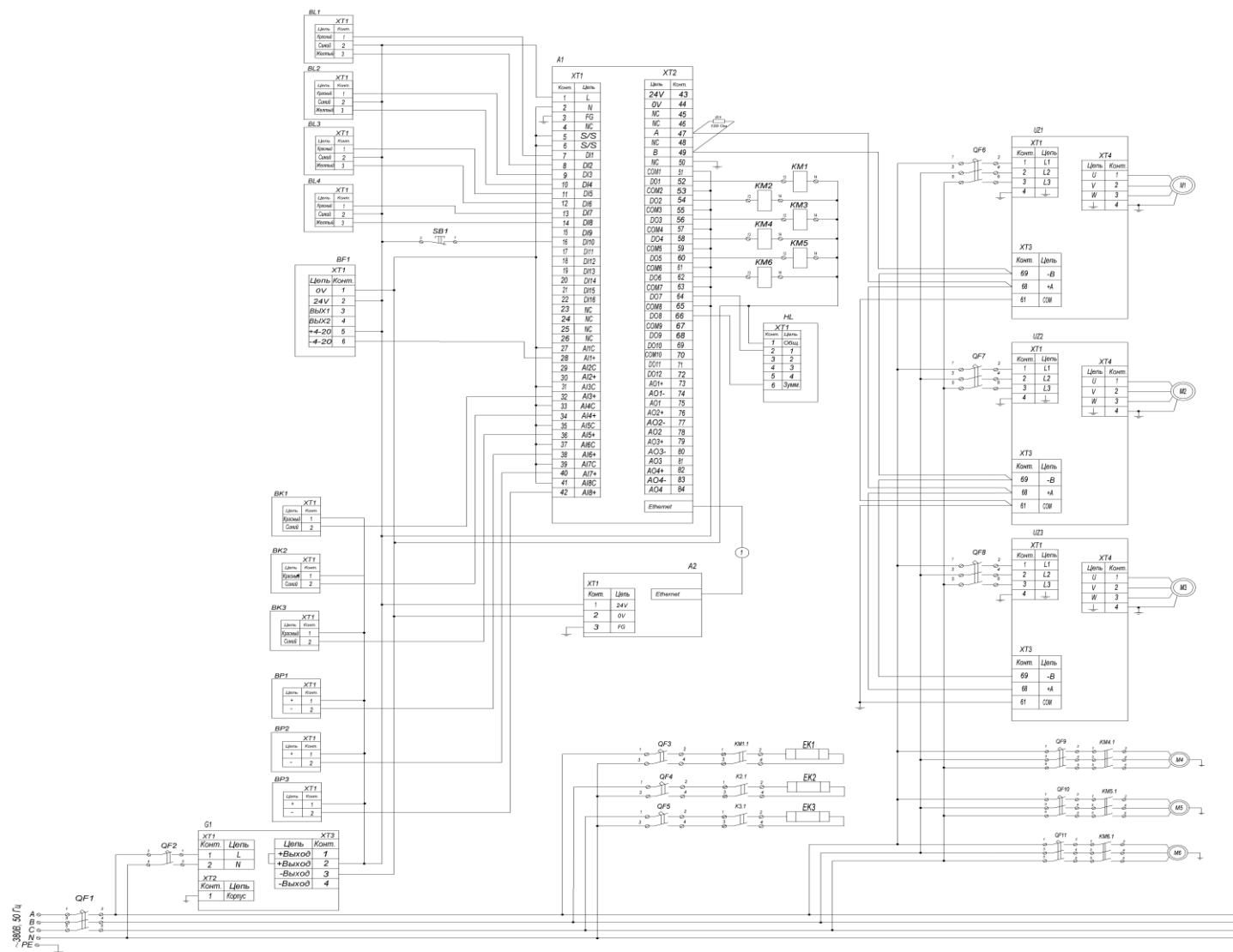
Рисунок 4.5 – Электрическая схема подключения
