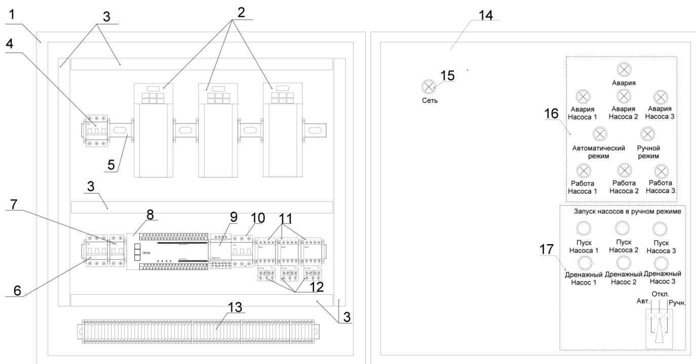
Рисунок 4.1 – Шкаф управления водозабором*:
